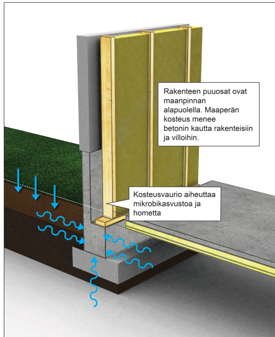
Perinteinen valesokkelirakenne
