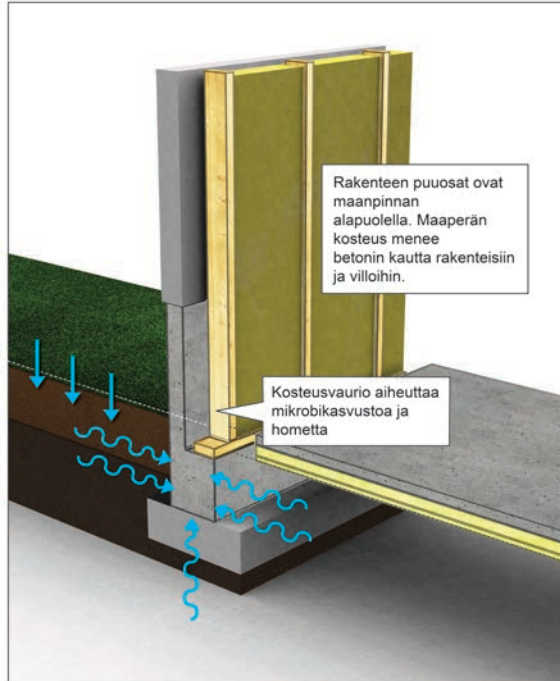
Perinteinen valesokkelirakenne
